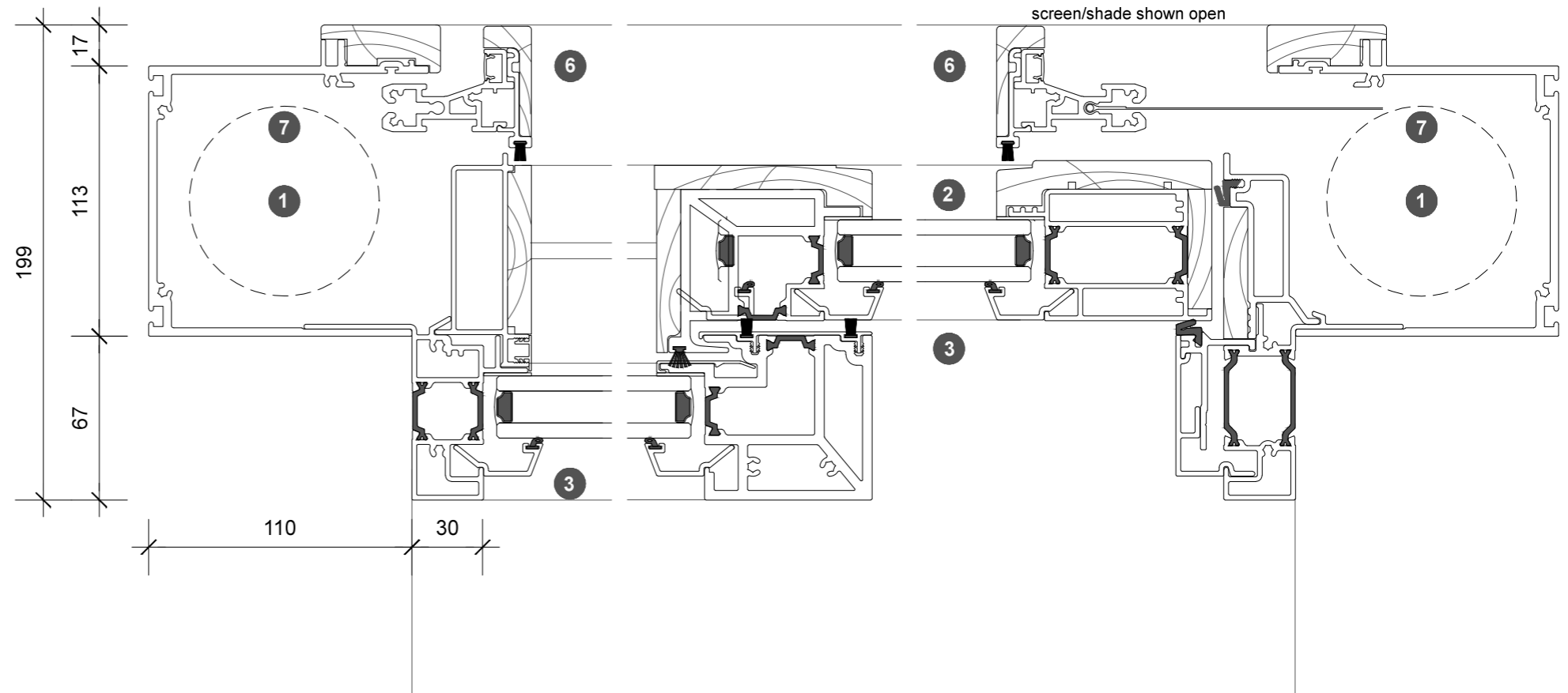
1. jamb detail
